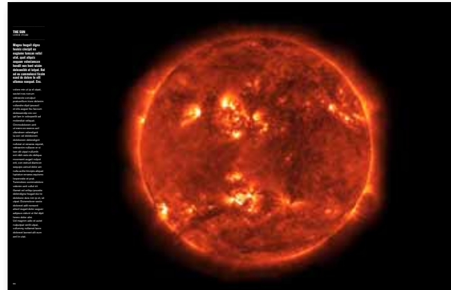
SUN
